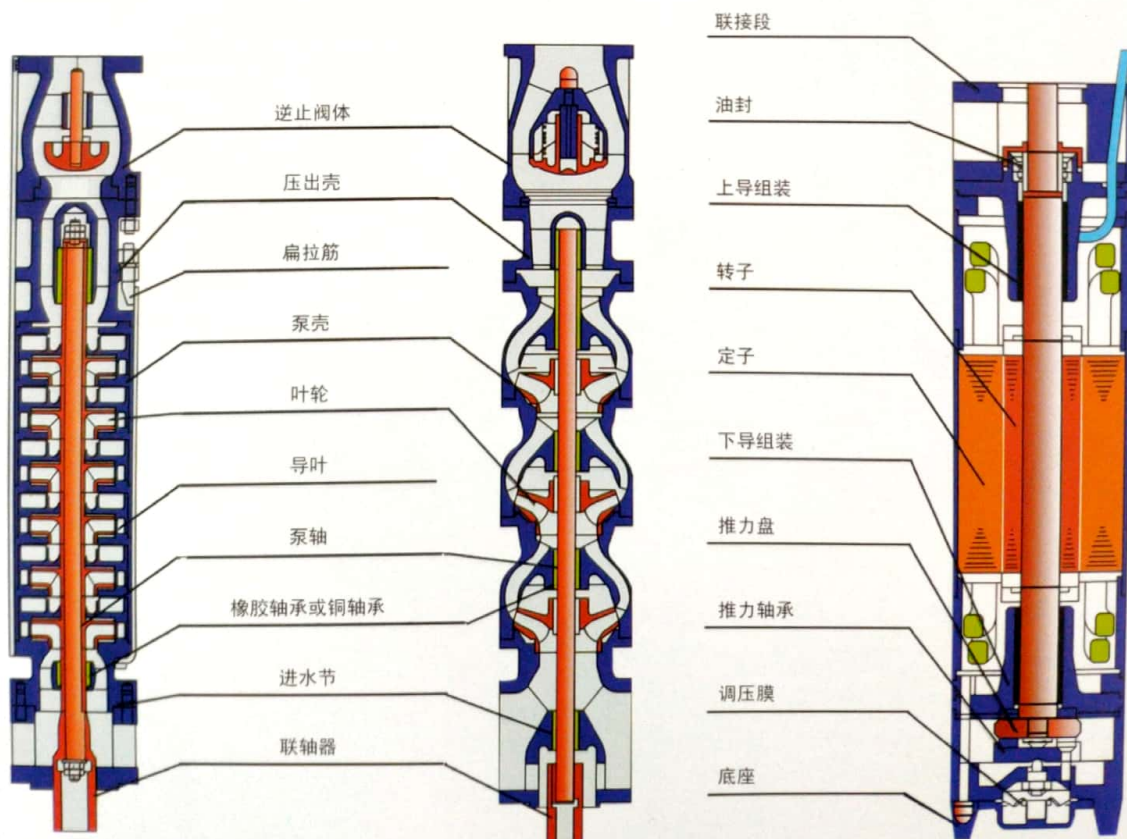
扁拉筋连接泵
