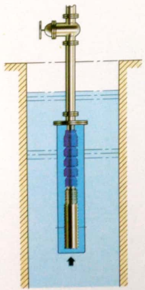
开放性水域立式安装结构图
