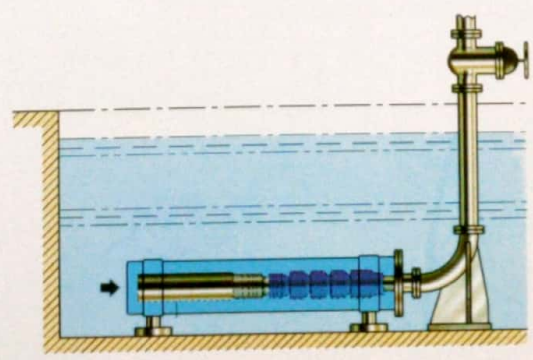
开放性水域卧式安装结构图
